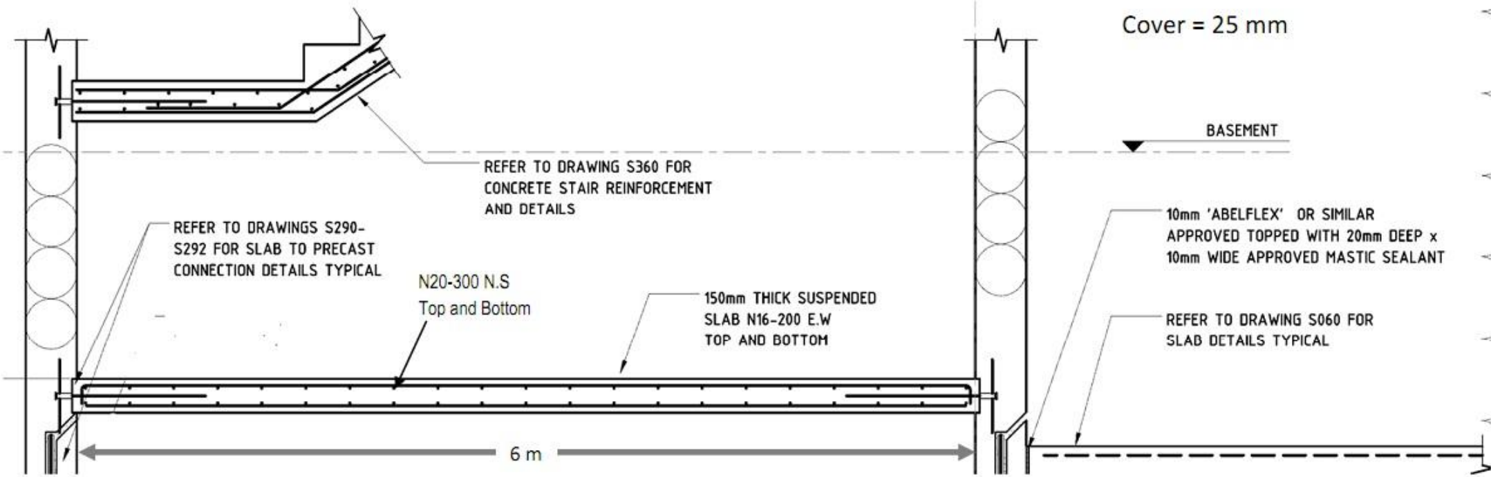
SECTION A-A
